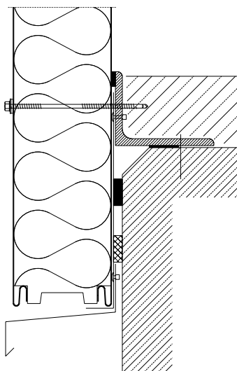
onderdetail horizontale montage
